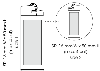
BIC® J23: (2,2 cm W x 7,6 cm H x 1,1 cm D)
